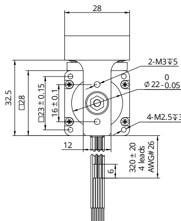
DS-DLG 28
