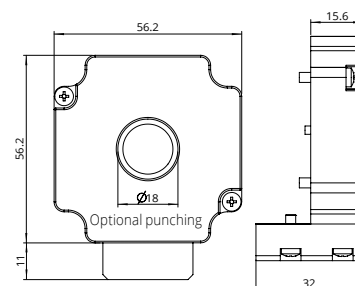
EK 4 Encoder 23
