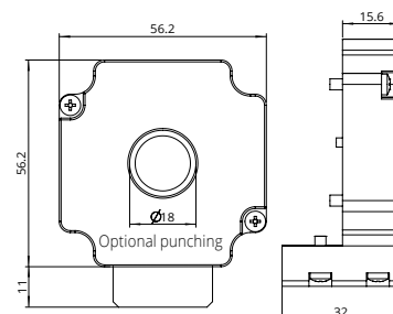
EK 4 Encoder 23
