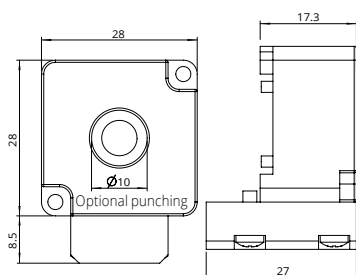
EK 4 Encoder 11
